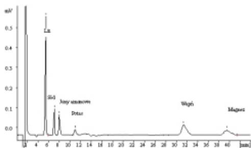
Rys. 4 Chromatogram rozdzielania wybranych nieorganicznych kationów.
