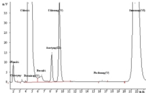
Rys. 2 Chromatogram próbki dezynfekowanej wody z basenu kąpielowego
