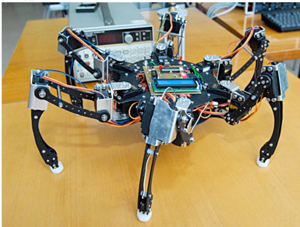
TriHex wyposażony jest w 18 napędów i porusza się w sposób trójpodporowy.
